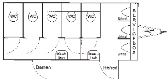
Raumeinteilung WC-Anhänger 5 m
